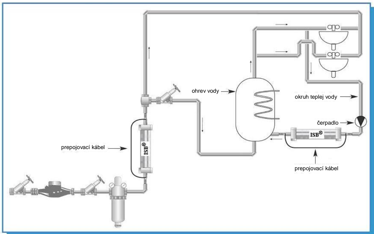
Inštalácia na vstupe studenej vody a v cirkulačnom okruhu teplej vody
